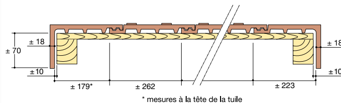
RABAT DROIT ET RABAT GAUCHE (Uniquement pour la tuile Actua)
