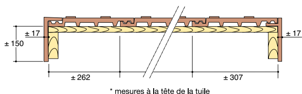
POSE AVEC RIVES INDIVIDUELLES GAUCHE ET DROITE Utiliser une demi-tuile un rang sur deux
