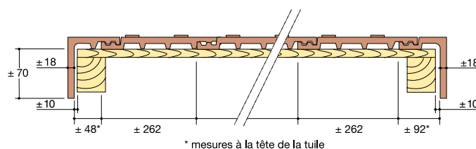
DEMI-RABAT DROIT ET DEMI-RABAT GAUCHE La tuile Actua Duplex ne se pose qu'avec des demi-rabats avec une demi-tuile un rang sur deux
