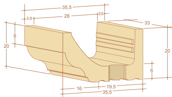
Corniche CO (doucine)
