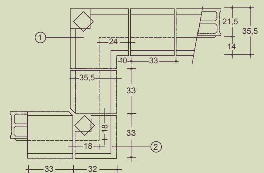
Schéma d'assemblage CO / CC
