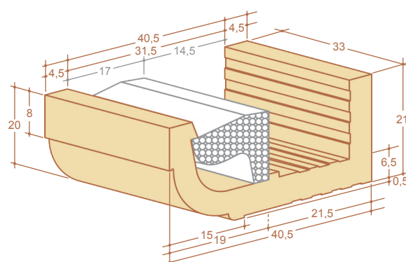
Corniche CR (quart de rond)
