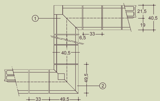
Schéma d'assemblage CR / CG
