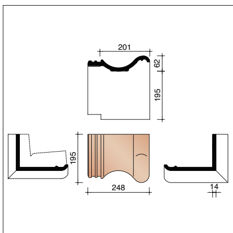
P4018500 5 pièces/m crt Tuile faîtière (collée)
