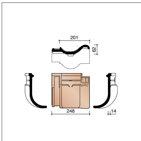
P4018200 5 pièces/m crt Tuile membron
