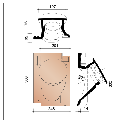
P4018741 Kit tuile à douille Ø 100 mm + mitron (95 cm 2 ) module de connexion + pièce de réductrice
