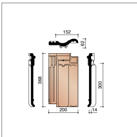
P4018030 3,4 pièces/m crt Tuile trois quart
