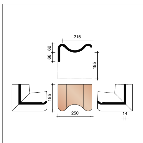
P4017580 Tuile faîtière de rive gauche (collée)
