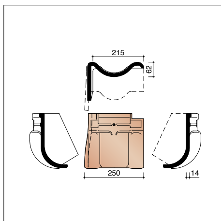
P4017280 Tuile membron de rive gauche
