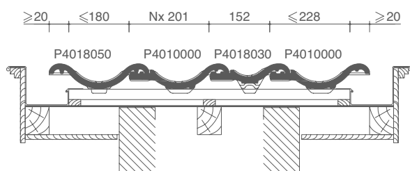
PLAN DE POSE LONGITUDINALE DE LA TOITURE AU NIVEAU DE LA TUILE FAÎTIÈRE
