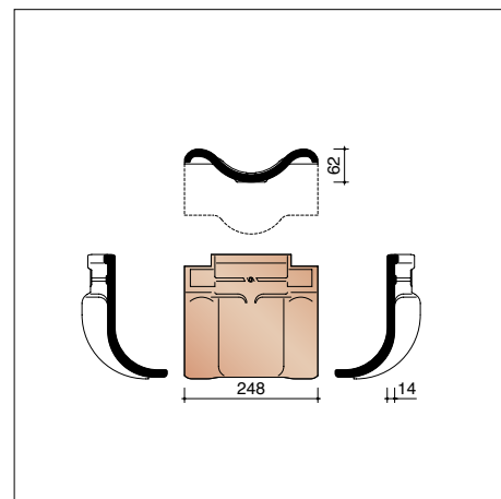
P4018250 Tuile membron à double bourrelet
