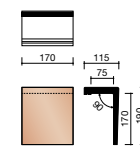
P301 8520 ① ② Tuile faitière 90° (5,9 au ml)
