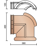
P000 5120 ☉ ☉ Rencontre 2 faîtières demi-rondes 230 mm et 1 arêtier demi-ronde 190 mm
