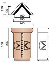
P000 0700 ☉ ☉ Faîtière "type église" avec crête et écusson (3,0 au ml)
