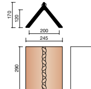
P000 0100 ☉ ☉ Faîtière spéciale avec 'coup de pouce' ancien modèle (3,4 au ml)
