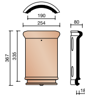
P000 3100 ☉ Arêtier demi-ronde 190 mm (3,0 au ml)
