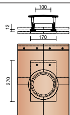
P301 8961 ① Kit tuile à douille Ø 100 mm
