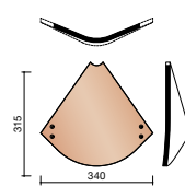
P301 3180 ① ② Noue imbriquée à 45° (9,1 au ml)
