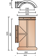
P000 5020 ☉ ☉ Rencontre 3 faîtières demi-rondes 230 mm
