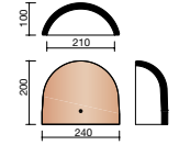
P000 3360 ☉ ☉ About d'arêtier demi-ronde sans emboîtement 210 mm
