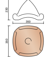
P000 5630 ☉ ☉ Rencontre 4 arêtiers demi-ronds 190 mm sans porte-boule
