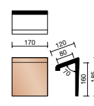
P301 8510 ① ② Tuile faitière 70° (5,9 au ml)
