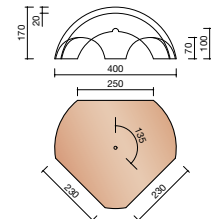
P000 5740 ☉ Jonction 1 faîtière demi-ronde 230 mm et 2 arêtiers demi-ronds 190 mm
