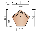
P000 0540 ☉ ☉ Plaque de rive avec bourrelet pour faîtière église
