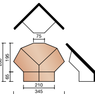
P000 5810 ① Rencontre 1 faitière angulaire et 2 arêtiers angulaires ou cornier
