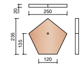
P000 0510 ☉ ☉ Plaque de rive à emboîtement pour faîtière église
