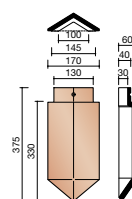
P000 3410 ① About d'arêtier angulaire à emboîtement
