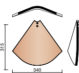
P301 3480 ① ② Arêtier imbriqué 45° (9,1 au ml)
