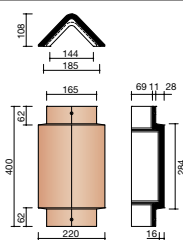
P000 1830 Faitière angulaire à double emboîtement
