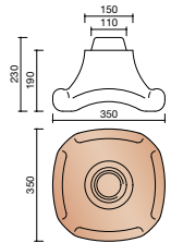
P000 5640 ☉ ☉ Rencontre 4 arêtiers demi-ronds 190 mm avec porte-boule
