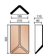
P000 5850 ① Rencontre 1 faitière angulaire et 2 arêtiers imbriqués
