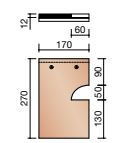
P301 8620 ① ② Tuile sous-chatière gauche
