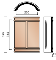
P000 1230 ☉ Faîtière demi-ronde 230 mm à double emboîtement
